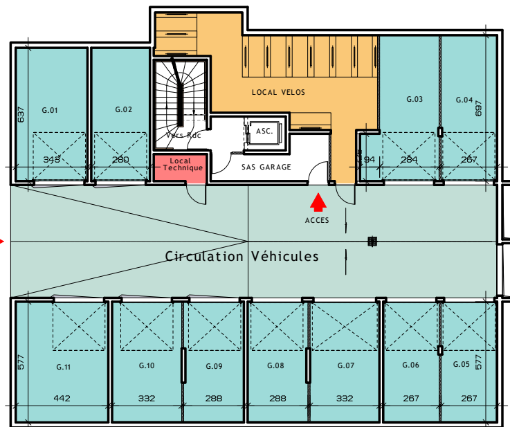
NIVEAU R-1
