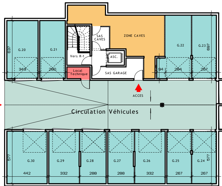
NIVEAU R-2
