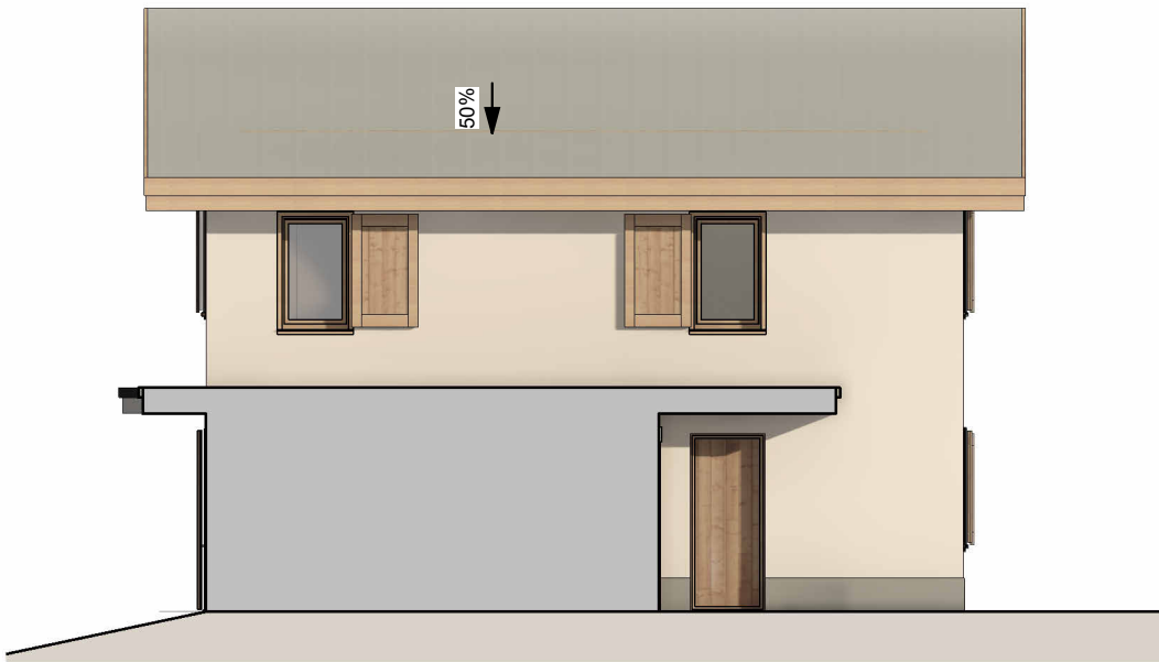
4 PDV - Maison 8 - Façade Nord-Est Ech : 1 : 100
