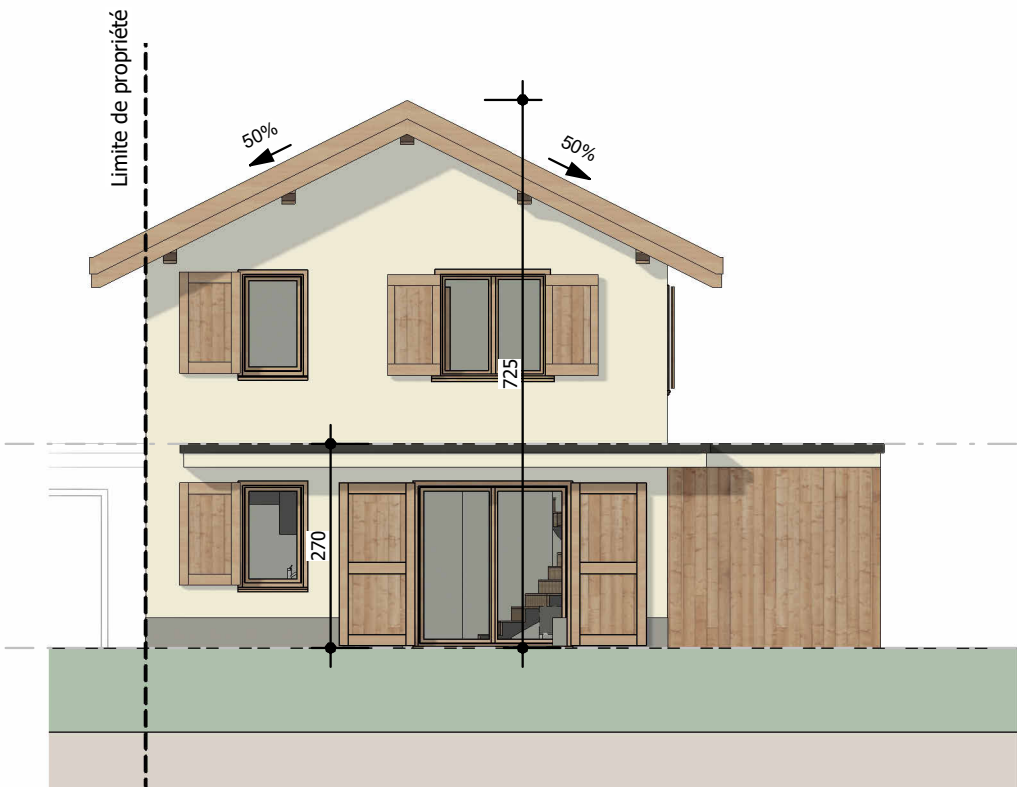
1 PDV - Maison 9 - Façade Sud-Est Ech : 1 : 100
