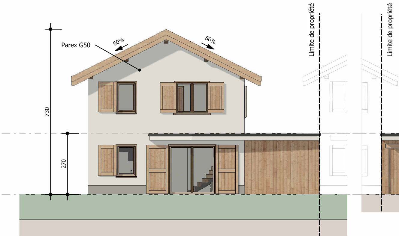
1 PDV - Maison 6 - Façade Sud-Est Ech : 1 : 100
