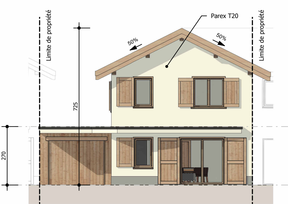
1 PDV - Maison 4 - Façade Sud Ech : 1 : 100
