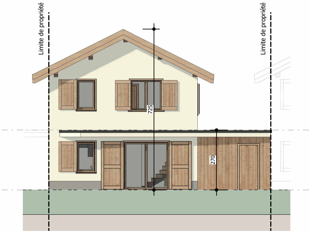
1 PDV - Maison 7 - Façade Sud-Est Ech : 1 : 100
