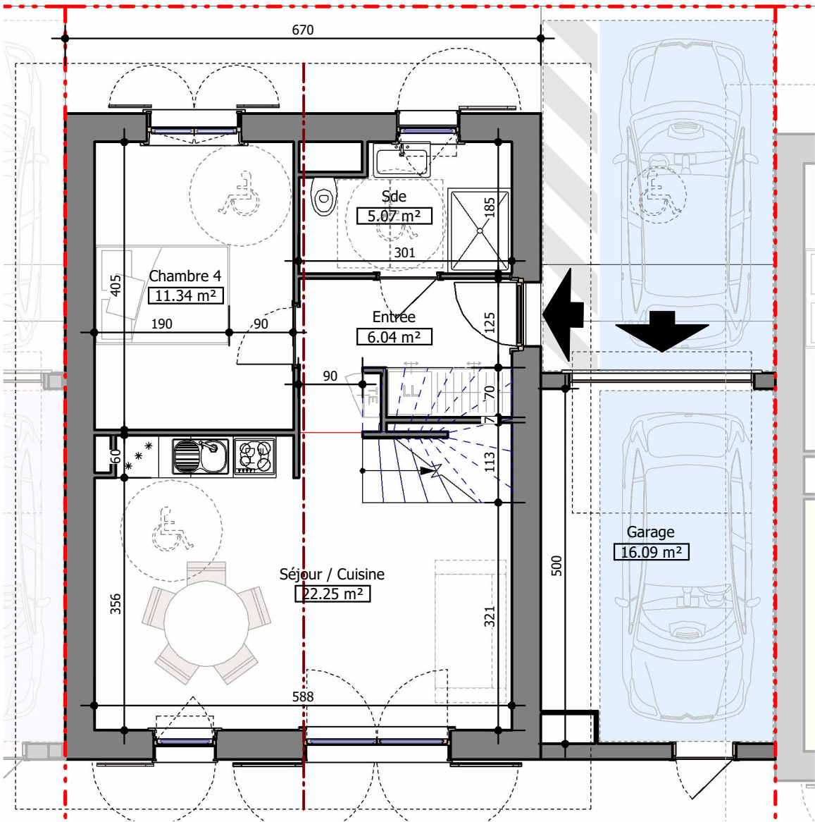
1 PDV - Maison 8 - Niveau 0 Ech : 1 : 75
