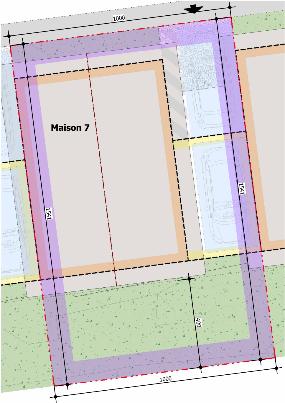
2 PDV - Plan Masse - M7 Ech : 1 : 100
