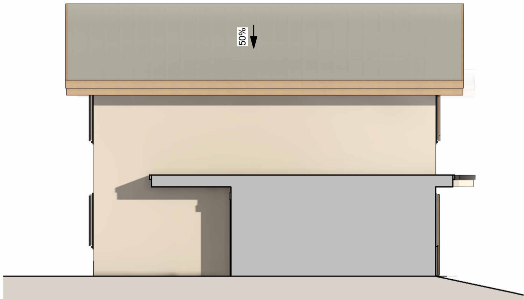
3 PDV - Maison 8 - Façade Sud-Ouest Ech : 1 : 100
