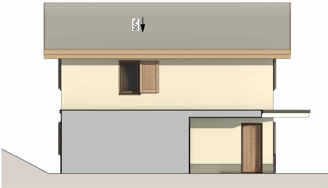
3 PDV - Maison 2 - Façade Sud-Ouest Ech : 1 : 100
