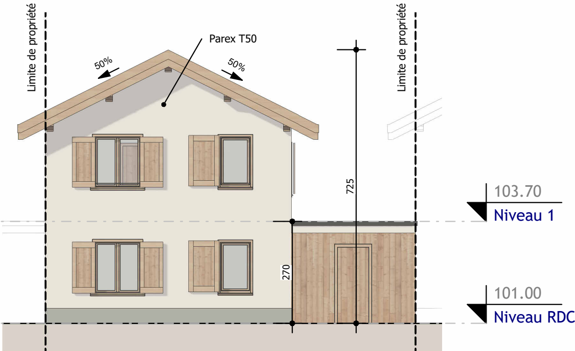
2 PDV - Maison 3- Façade Nord-Ouest Ech : 1 : 100
