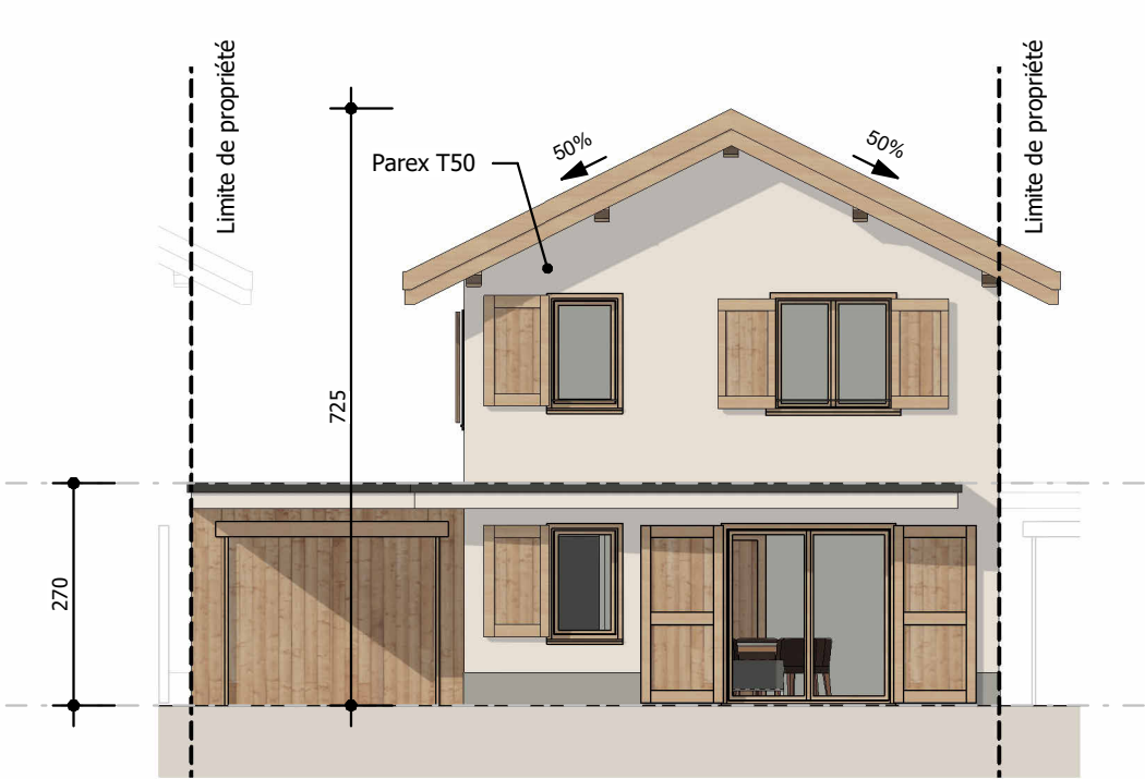
1 PDV - Maison 3 - Façade Sud-Est Ech : 1 : 100
