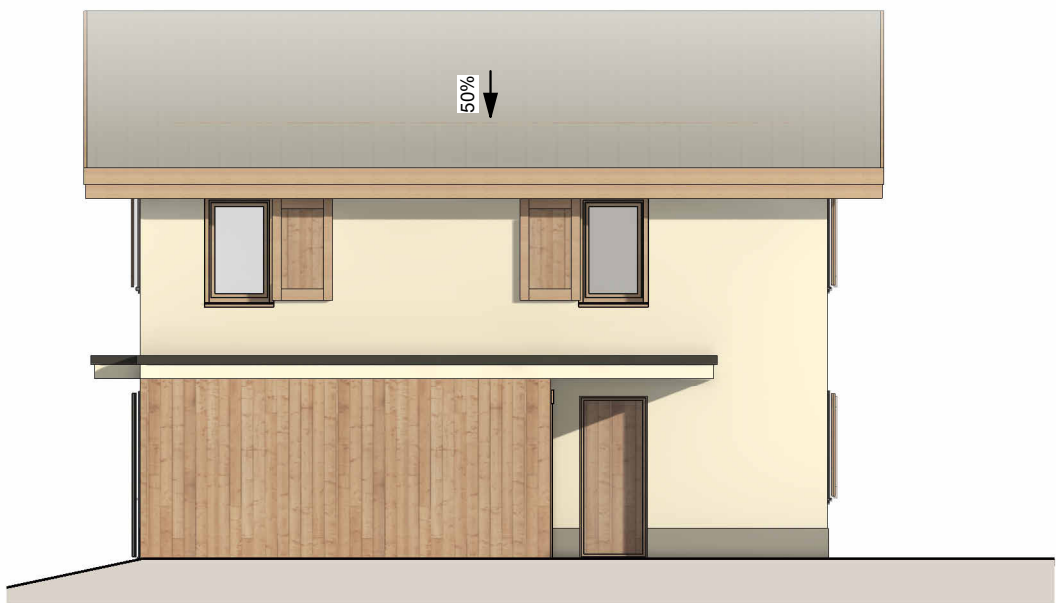
4 PDV - Maison 9 - Façade Nord-Est Ech : 1 : 100
