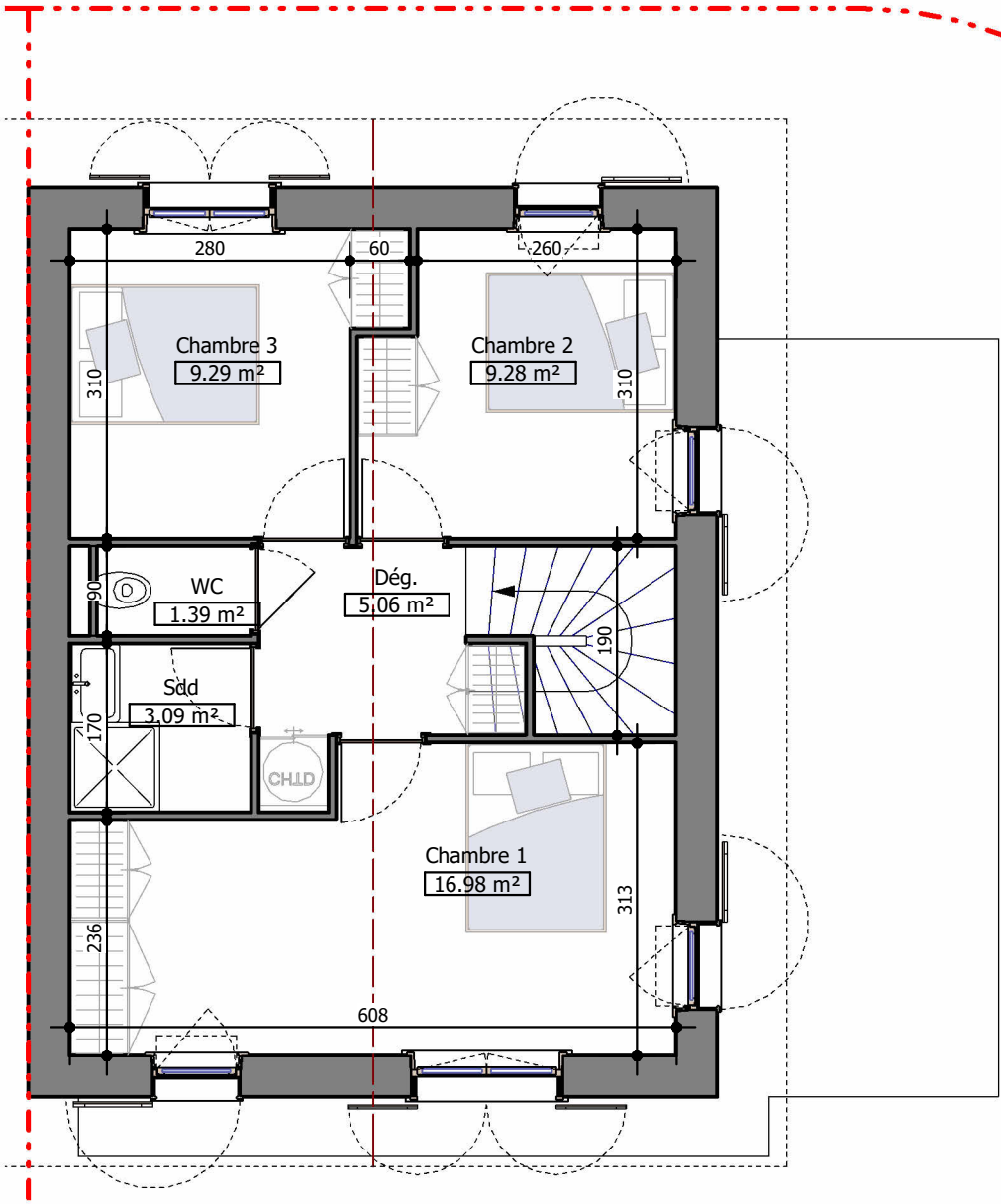
3 PDV - Maison 9 - Niveau 1 Ech : 1 : 75
