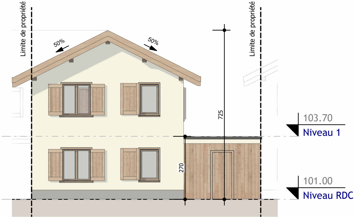
2 PDV - Maison 4- Façade Nord-Ouest Ech : 1 : 100
