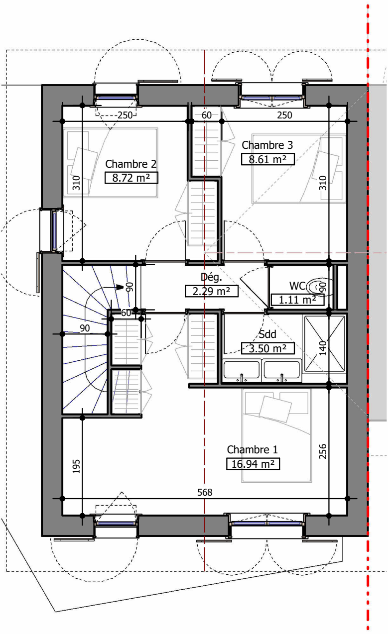
2 PDV - Maison 4 - Niveau 1 Ech : 1 : 75
