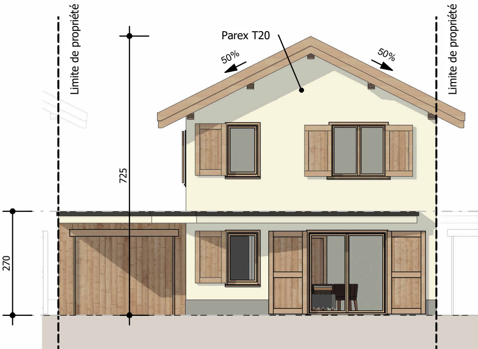
1 PDV - Maison 2 - Façade Sud-Est Ech : 1 : 100
