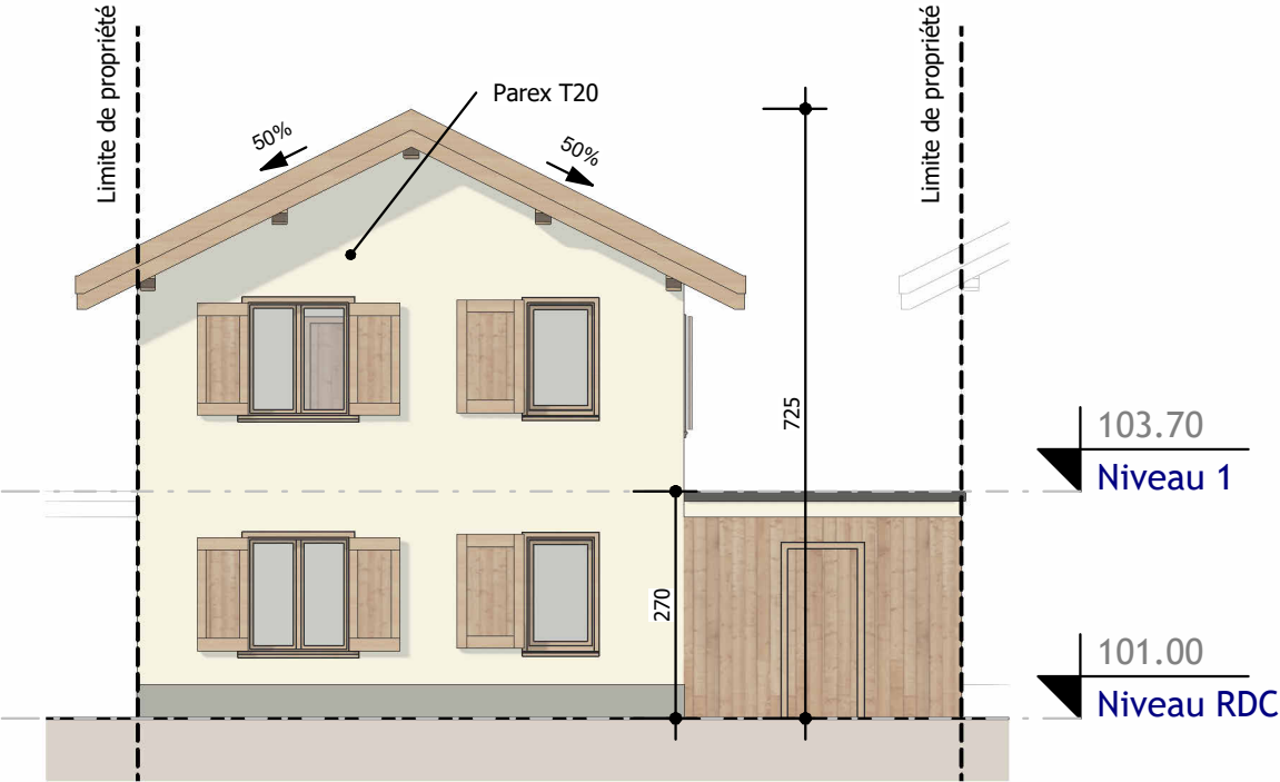
2 PDV - Maison 2- Façade Nord-Ouest Ech : 1 : 100
