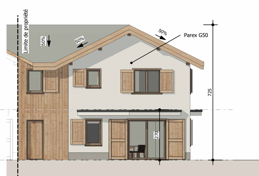
1 PDV - Maison 5 - Façade Sud Ech : 1 : 100
