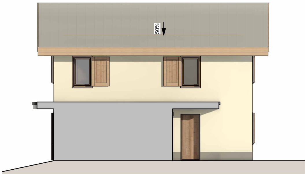
4 PDV - Maison 7 - Façade Nord-Est Ech : 1 : 100
