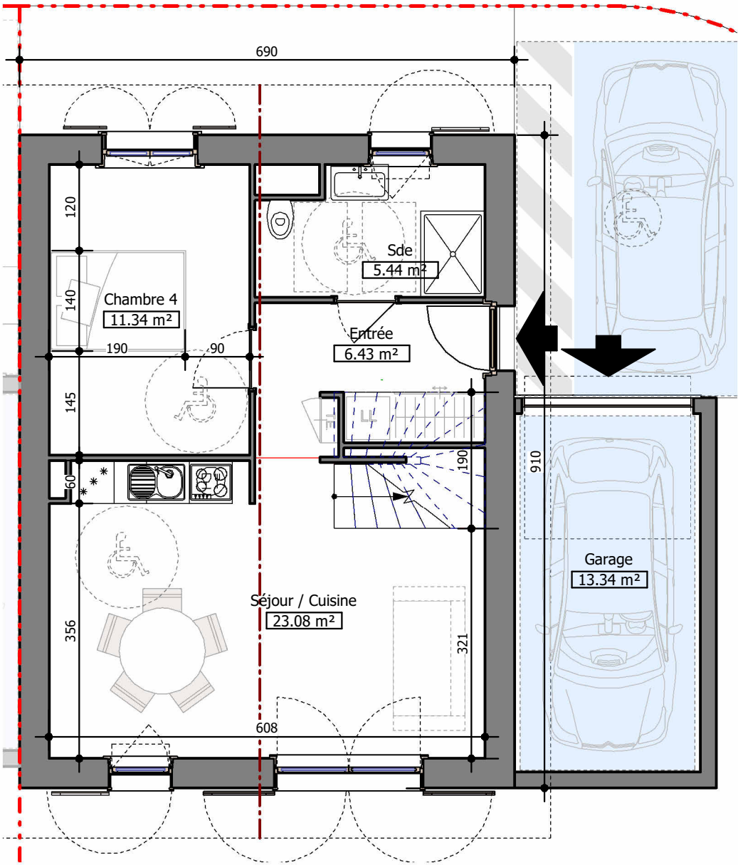
1 PDV - Maison 9 - Niveau 0 Ech : 1 : 75
