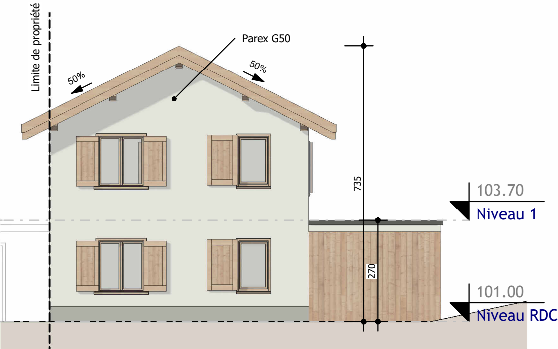
2 PDV - Maison 1- Façade Nord-Ouest Ech : 1 : 100
