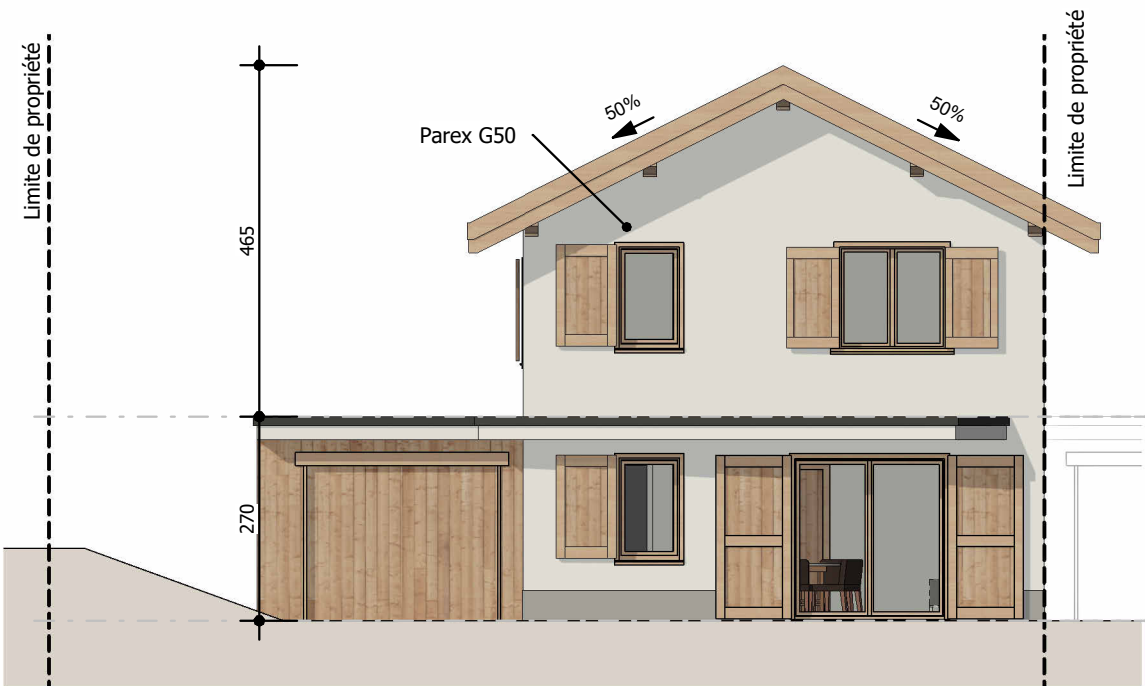
1 PDV - Maison 1 - Façade Sud-Est Ech : 1 : 100
