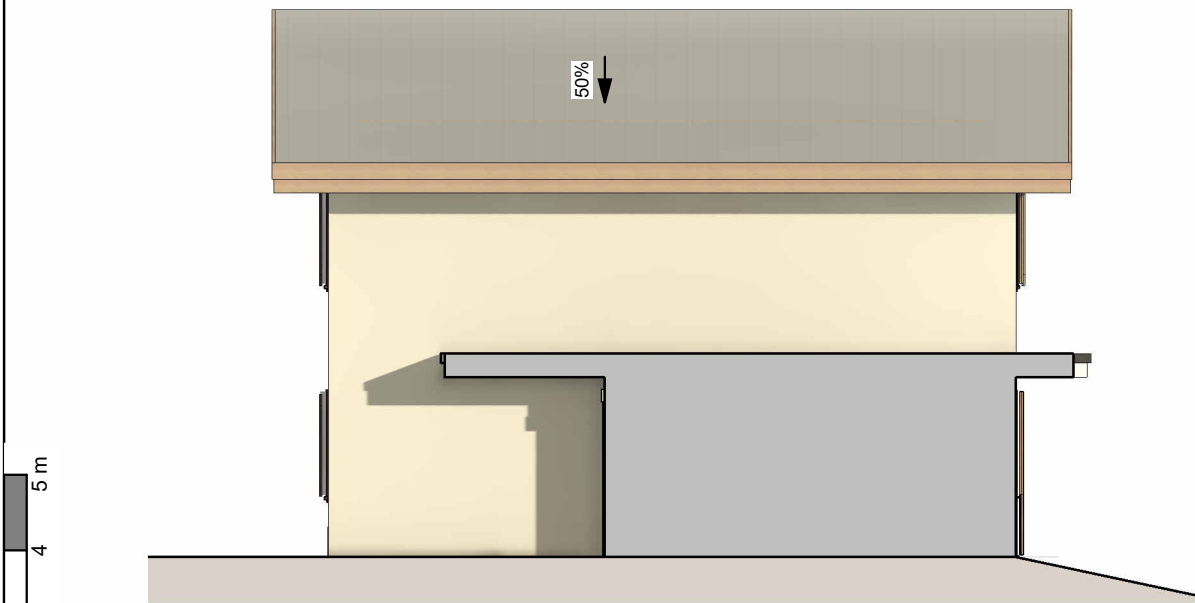
3 PDV - Maison 7 - Façade Sud-Ouest Ech : 1 : 100
