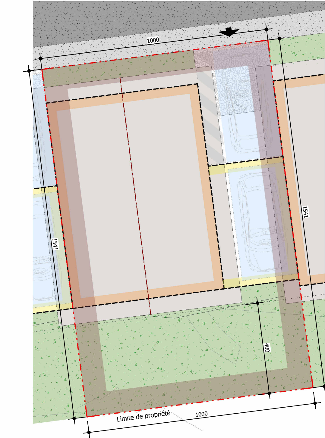
2 PDV - Plan Masse - M8 Ech : 1 : 100
