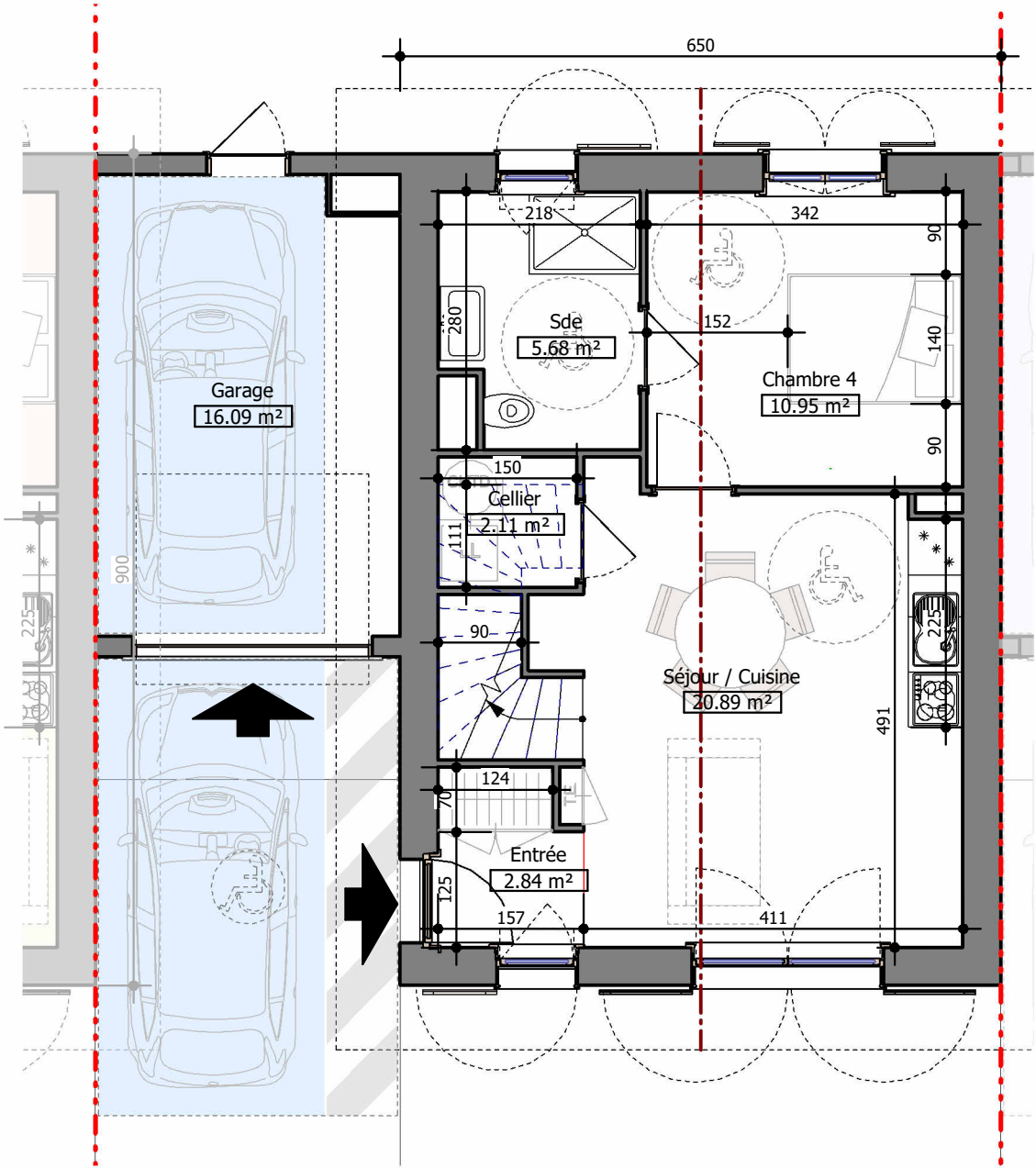
1 PDV - Maison 2 - Niveau 0 Ech : 1 : 75
