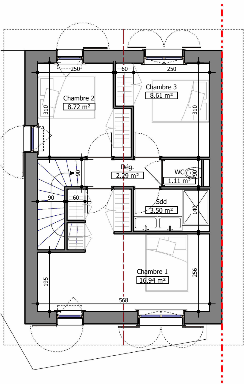
2 PDV - Maison 2 - Niveau 1 Ech : 1 : 75
