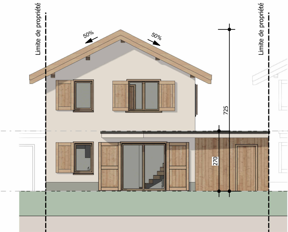
1 PDV - Maison 8 - Façade Sud-Est Ech : 1 : 100
