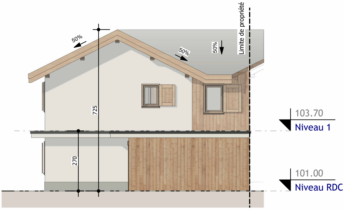
2 PDV - Maison 5- Façade Nord-Ouest Ech : 1 : 100
