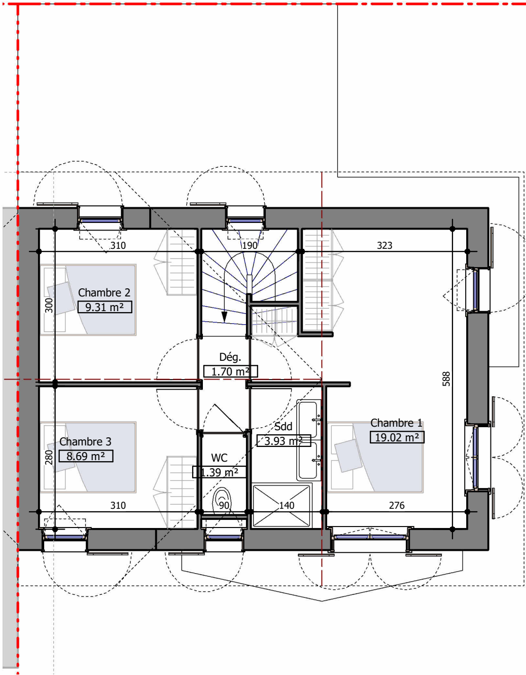
2 PDV - Maison 5 - Niveau 1 Ech : 1 : 75
