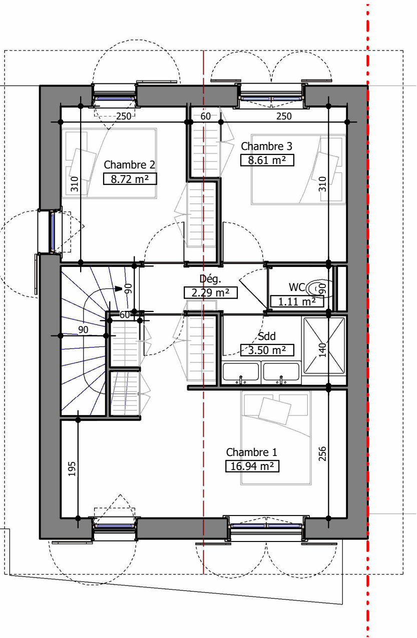
2 PDV - Maison 3 - Niveau 1 Ech : 1 : 75
