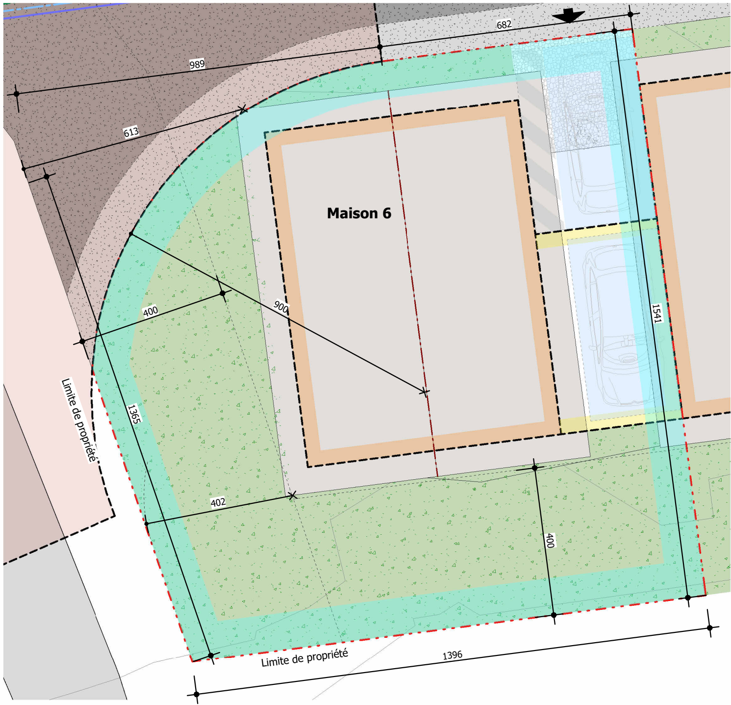
1 PDV - Plan Masse - M6 Ech : 1 : 100
