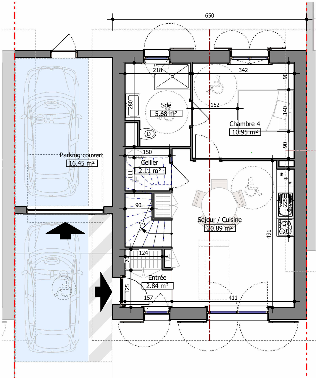
1 PDV - Maison 4 - Niveau 0 Ech : 1 : 75
