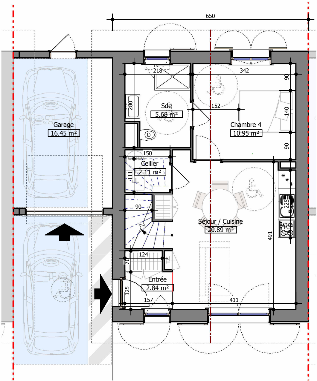
1 PDV - Maison 3 - Niveau 0 Ech : 1 : 75
