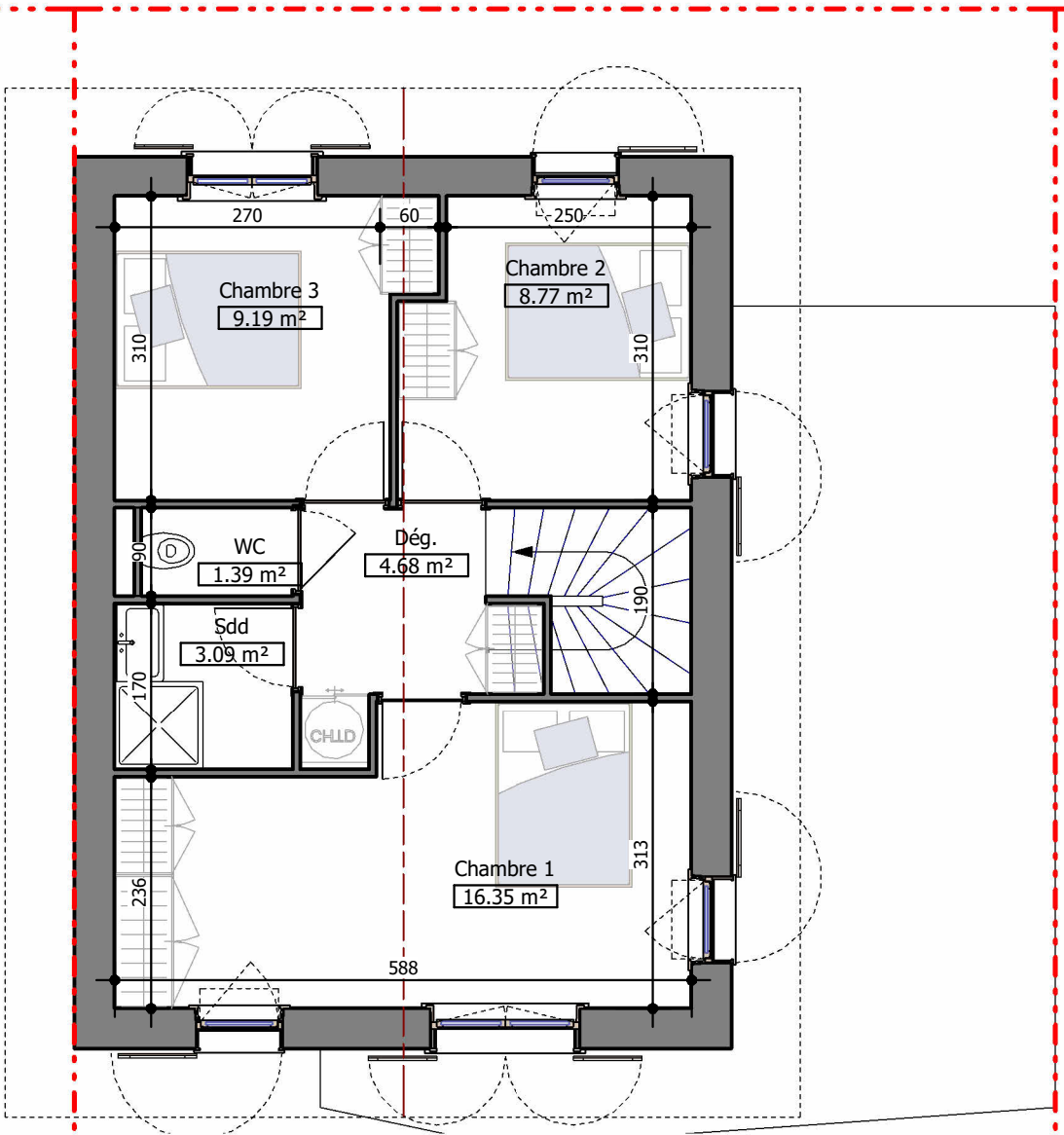
2 PDV - Maison 8 - Niveau 1 Ech : 1 : 75
