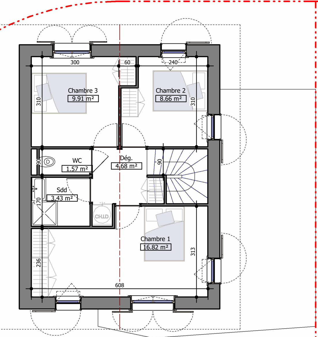
2 PDV - Maison 6 - Niveau 1 Ech : 1 : 75
